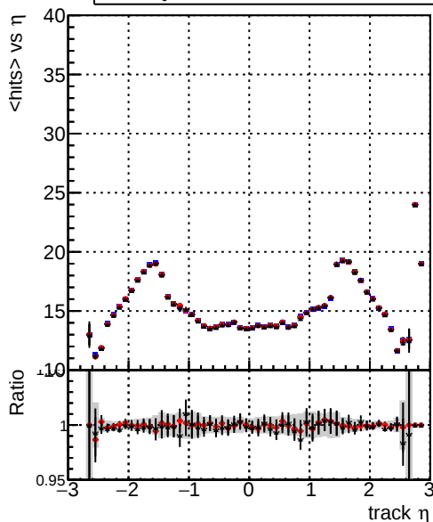
mean hits — DQM_mkFit_TToriginal — DQM_mkFit_TTNEUHS_ALLITERS — DQM_mkFit_TTNEUHSMS_ALLITERS
