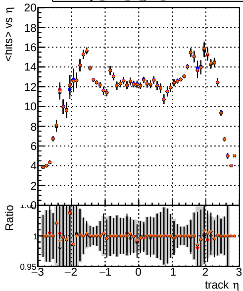
mean hit DQM_mkFit TT original DQM_mkFit TT pL DQM_mkFit TT pLW DQM_mkFit TT pLW IMP
