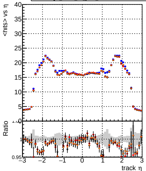
DQM_mkFit TT original DQM_mkFit TT pL DQM_mkFit TT pLW DQM_mkFit TT pLW IMP
