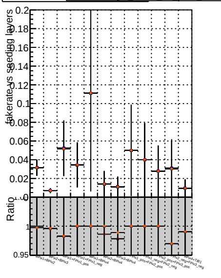
Fake rate vs. Original BGM mkFit BGM mkFit + BEW IMP
