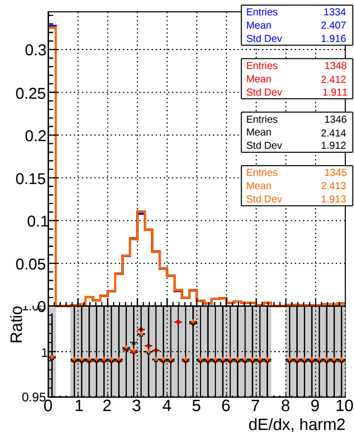
dE/dx estimator 1
