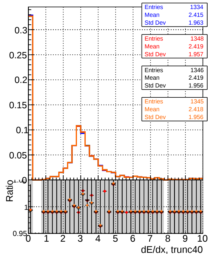
dE/dx estimator 2
