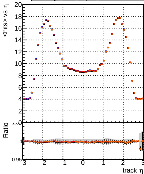
mean hit DOM_mkFit TT original DOM_mkFit TT pL DOM_mkFit TT pLW DOM_mkFit TT pLW IMP
