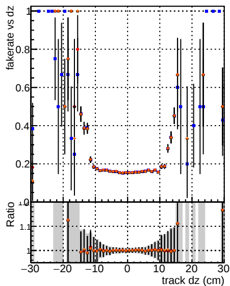
DQM mkFit T Original DQM mkFit T BEW IMP
