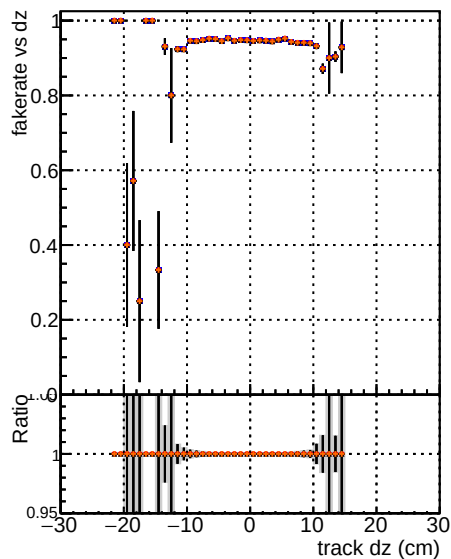
Fake rate vs dz BGM mkt fit Toriginal BGM mkt fit BEW 1H
