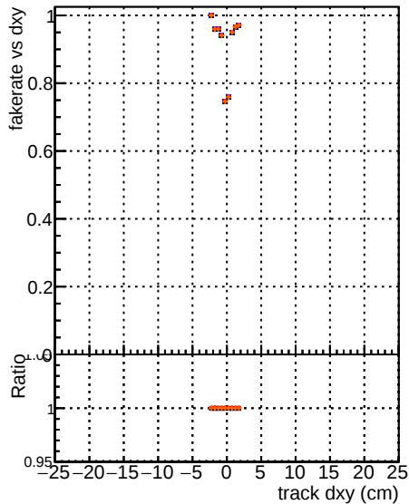
Fake rate vs d DSM mkFit Toriginal DSM mkFit TBEW 1H DSM mkFit Toriginal DSM mkFit TBEW 1H
