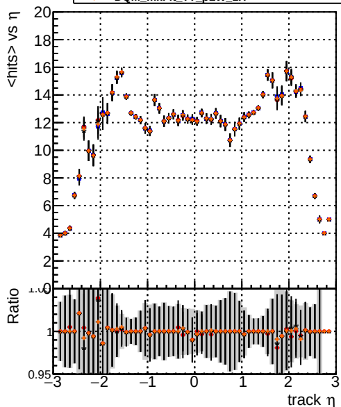
Legend: — DQM_mkFit TT original — DQM_mkFit TT pL — DQM_mkFit TT pLW — DQM_mkFit TT pLW_1H mean hit
