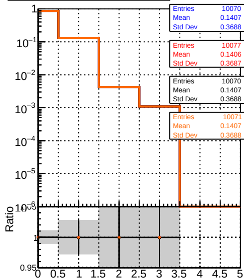
Legend: — DQM_mkFit TT original — DQM_mkFit TT pL — DQM_mkFit TT pLW — DQM_mkFit TT pLW_1H mean hit
