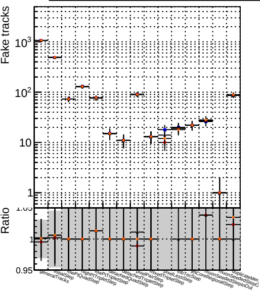
Number ■ DQM mkFit TT original ● DQM mkFit TT pL ▲ DQM mkFit TT pLW ◆ DQM mkFit TT pLW 1H
