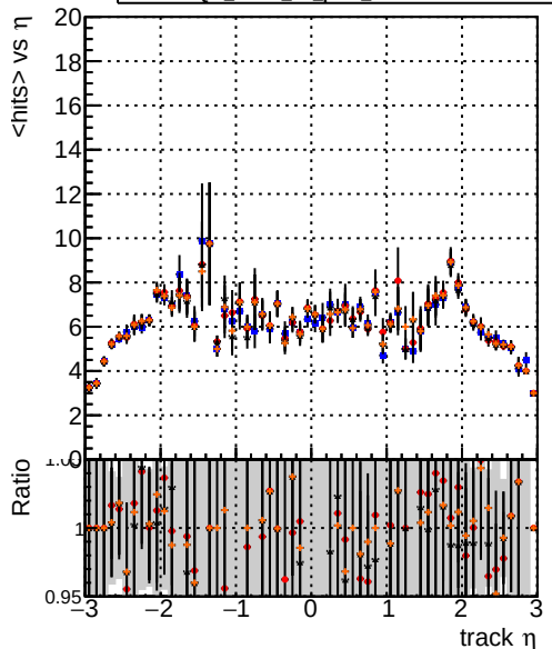
— DQM_mkFit TT original — DQM_mkFit TT pL — DQM_mkFit TT pLW — DQM_mkFit TT pLW 1H
