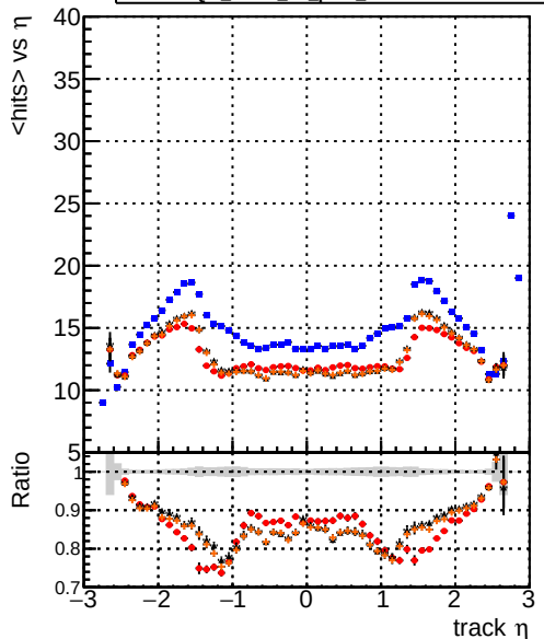
— DQM_mkFit TT original — DQM_mkFit TT pL — DQM_mkFit TT pLW — DQM_mkFit TT pLW 1H mean hits
