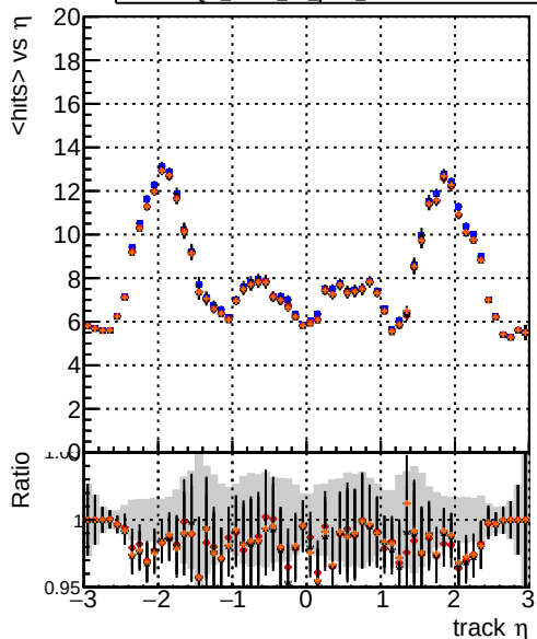
mean hit DQM_mkFit TT original DQM_mkFit TT pL DQM_mkFit TT pLW DQM_mkFit TT pLW 1H
