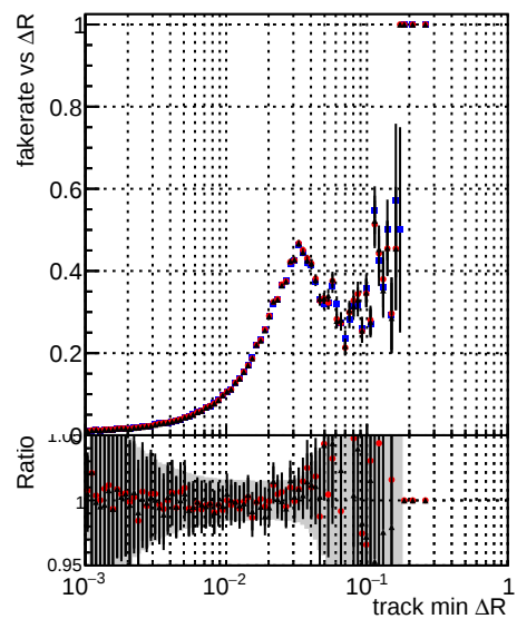
—●— DQM mkFit TT original —●— DQM mkFit TT pL —●— DQM mkFit TT pLW
