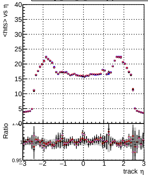
mean hits DQM mkFit TT original DQM mkFit TT newStudy DQM mkFit TT newStudy4 DQM mkFit TT newStudyhp4
