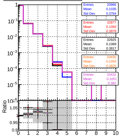
mean hits DQM mkFit TT original DQM mkFit TT newStudy DQM mkFit TT newStudy4 DQM mkFit TT newStudy4h DQM mkFit TT newStudy4hp4
