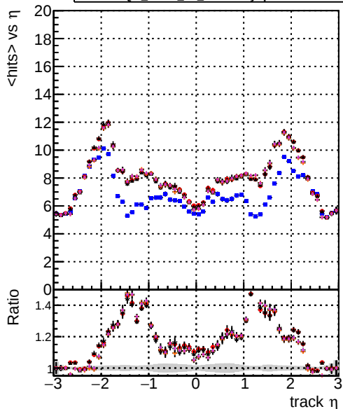
mean hit DQM mkFit TT original DQM mkFit TT newStudy DQM mkFit TT newStudy4 DQM mkFit TT newStudy4h DQM mkFit TT newStudy4hp4
