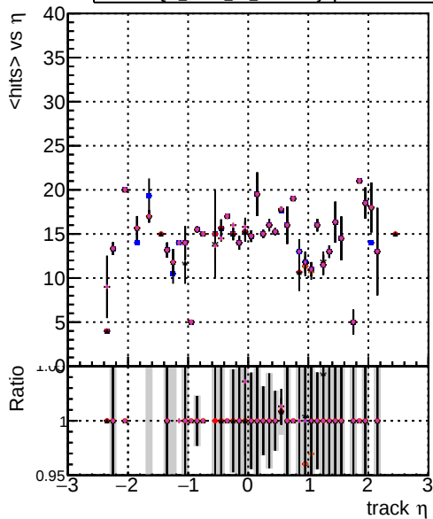
mean hit DQM mkFit TT original DQM mkFit TT newStudy DQM mkFit TT newStudyhp4 DQM mkFit TT newStudyhp4
