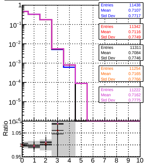
mean hits DQM mkFit TT original DQM mkFit TT newStudy DQM mkFit TT newStudy4 DQM mkFit TT newStudyh DQM mkFit TT newStudyhp4
