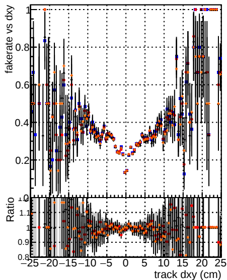
—●— DQM mktFit TTEFW TTEFW-improved —●— DQM mktFit TTEFW TTEFW-improved
