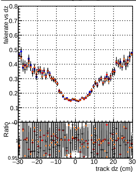
—●— DQM mktFit TTEFW TTEFW-improved —●— DQM mktFit TTEFW TTEFW-improved
