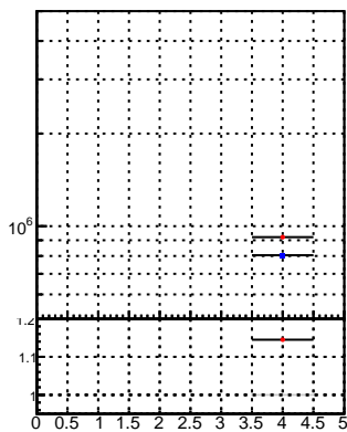
Fit_BDT_lowpT
