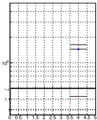
N of reco track vs la 0 0.00 1 0.00 2 0.00 3 0.00 4 0.00 5 0.00 6 0.00 7 0.00 8 0.00 9 0.00 10 0.00 11 0.00 12 0.00 13 0.00 14 0.00 15 0.00 16 0.00 17 0.00 18 0.00 19 0.00 20 0.00 21 0.00 22 0.00 23 0.00 24 0.00 25 0.00 26 0.00 27 0.00 28 0.00 29 0.00 30 0.00 31 0.00 32 0.00 33 0.00 34 0.00 35 0.00 36 0.00 37 0.00 38 0.00 39 0.00 40 0.00 41 0.00 42 0.00 43 0.00 44 0.00 45 0.00 46 0.00 47 0.00 48 0.00 49 0.00 50 0.00 51 0.00 52 0.00 53 0.00 54 0.00 55 0.00 56 0.00 57 0.00 58 0.00 59 0.00 60 0.00 61 0.00 62 0.00 63 0.00 64 0.00 65 0.00 66 0.00 67 0.00 68 0.00 69 0.00 70 0.00 71 0.00 72 0.00 73 0.00 74 0.00 75 0.00 76 0.00 77 0.00 78 0.00 79 0.00 80 0.00 81 0.00 82 0.00 83 0.00 84 0.00 85 0.00 86 0.00 87 0.00 88 0.00 89 0.00 90 0.00 91 0.00 92 0.00 93 0.00 94 0.00 95 0.00 96 0.00 97 0.00 98 0.00 99 0.00 100 0.00 101 0.00 102 0.00 103 0.00 104 0.00 105 0.00 106 0.00 107 0.00 108 0.00 109 0.00 110 0.00 111 0.00 112 0.00 113 0.00 114 0.00 115 0.00 116 0.00 117 0.00 118 0.00 119 0.00 120 0.00 121 0.00 122 0.00 123 0.00 124 0.00 125 0.00 126 0.00 127 0.00 128 0.00 129 0.00 130 0.00 131 0.00 132 0.00 133 0.00 134 0.00 135 0.00 136 0.00 137 0.00 138 0.00 139 0.00 140 0.00 141 0.00 142 0.00 143 0.00 144 0.00 145 0.00 146 0.00 147 0.00 148 0.00 149 0.00 150 0.00 151 0.00 152 0.00 153 0.00 154 0.00 155 0.00 156 0.00 157 0.00 158 0.00 159 0.00 16
