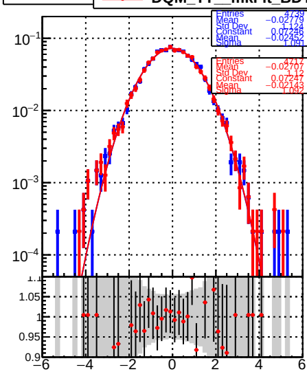
RecoPVAssoc
