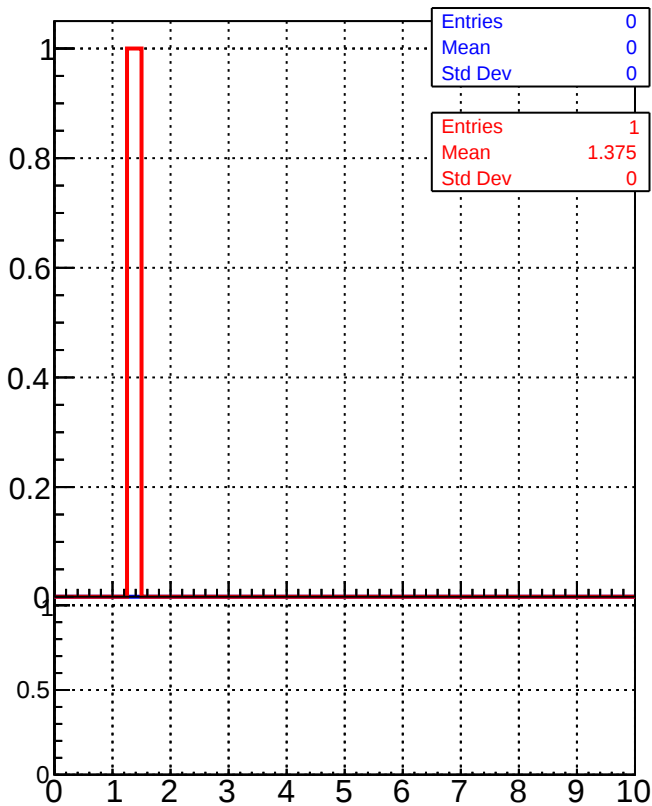
dE/dx estimator 1
