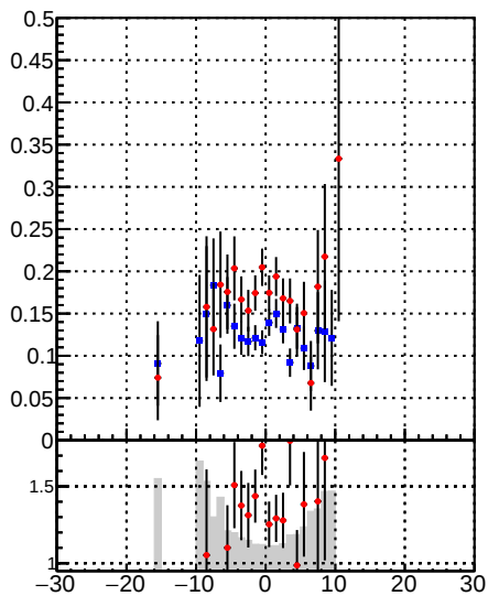
—●— DQM TT mkFit_lowpT —●— DQM TT mkFit_BDT_lowpT
