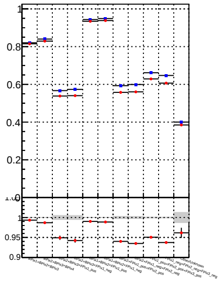
Fake rate vs. —●— DQM TT_mkFit_lowpT —●— DQM TT_mkFit_BDT_lowpT
