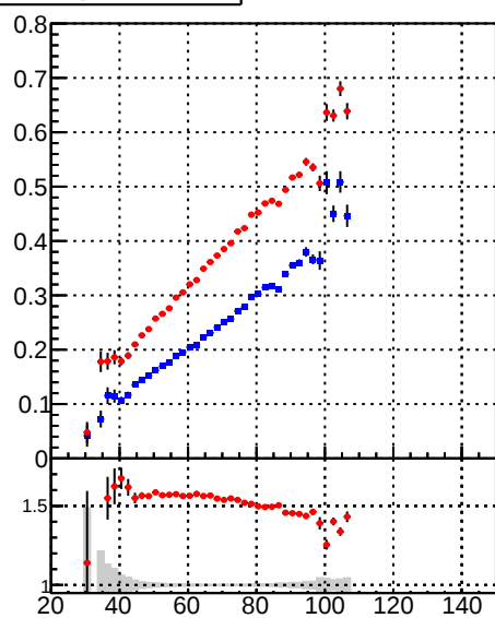
fake+duplicates vs PU
