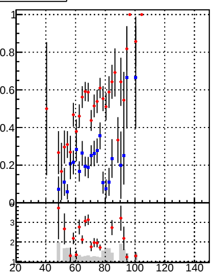
Fake rate vs pu
