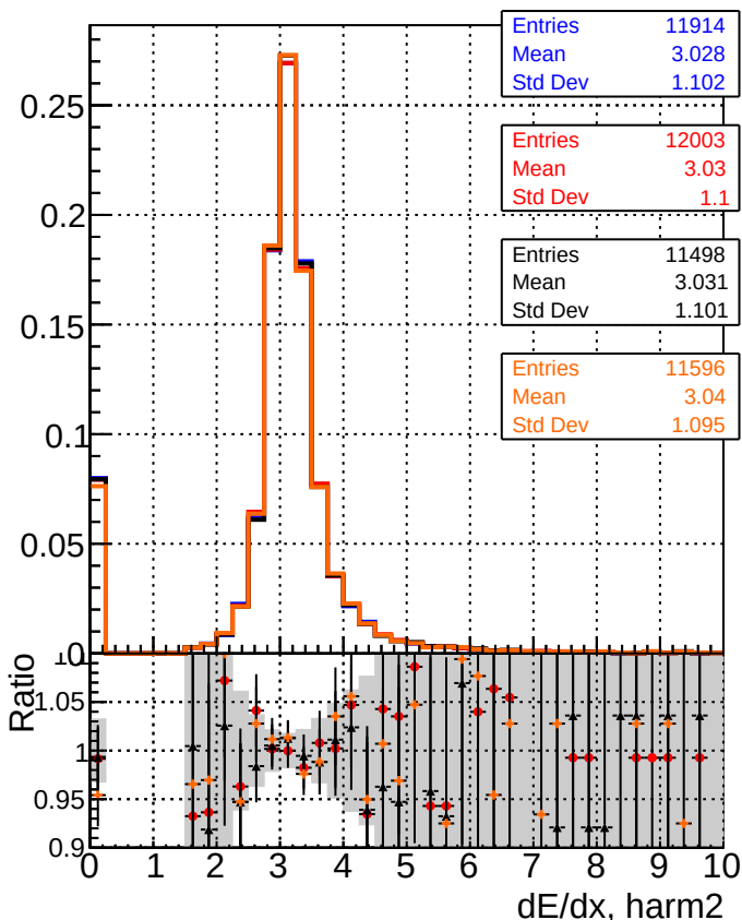
— DQM_mkFit TToriginal — DQM_mkFit TTNEWnoMS-genMatch-chi200 — DQM_mkFit TToriginal-106 — DQM_mkFit TTNEWMS-genMatch-chi200
