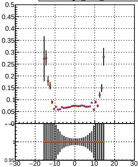
Legend for Fake rate vs v: DOM CKE DOM mKEit DOM BDT DOM mKEit CKEit
