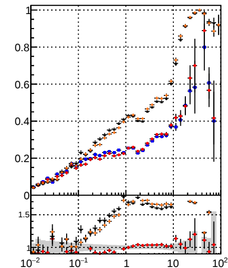
Legend for Fake rate vs vertpos: DOM CKE BDT mKEit BDT mKEit
