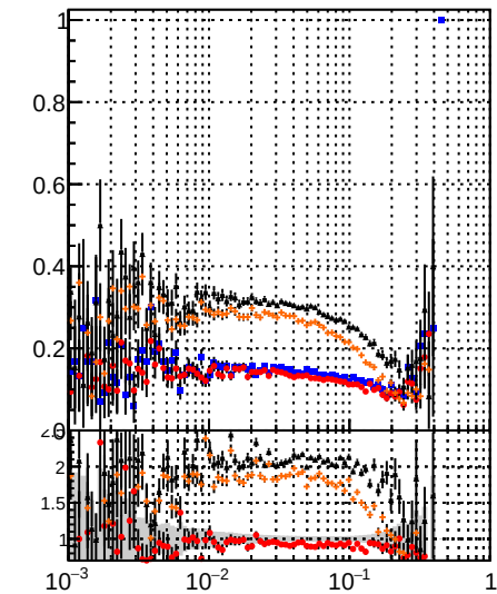
Fake rate vs \epsilon Legend: DOM CKE DOM mKEit DOM BDT BDT mKEit
