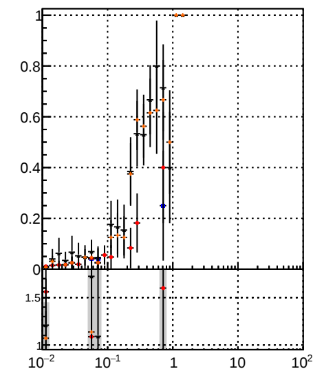
Fake rate vs v_z DOM CKE DOM mKEit DOM BDT mKEit
