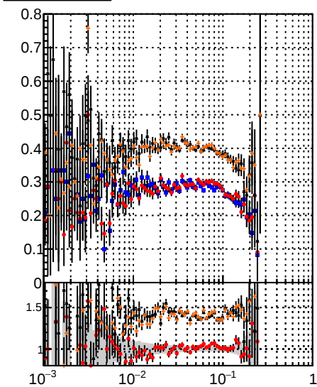
Fake rate vs \epsilon Legend: DOM CKE DOM mKEit DOM BDT DOM mKEit CKE
