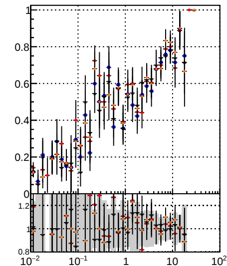
Fake rate vs \nu Legend: DOM CKE DOM mKEit DOM BDT CKE mKEit BDT
