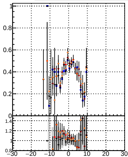
DOM CKE DOM mKEit DOM BDT CKEit Fake rate vs verpos
