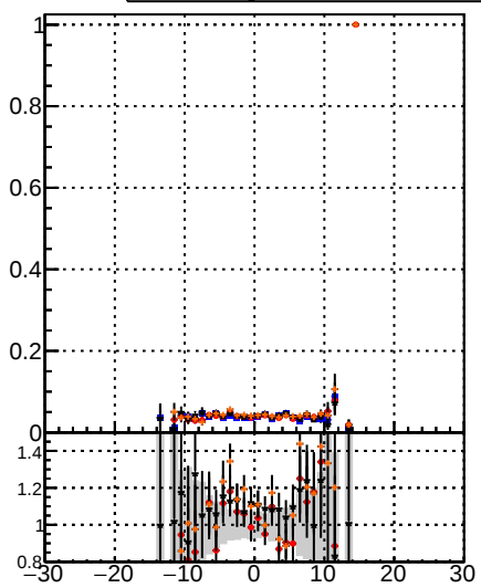
Fake rate vs v DOM CKE mKEit BDT mKEit
