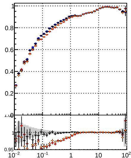
Legend for Fake rate vs v: DOM CKE DOM mKEit DOM BDT CKEit BDT mKEit
