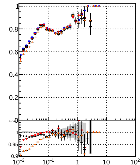
Legend for Fake rate vs vertpos: DOM CKE BDT mKEit BDT CKE BDT mKEit
