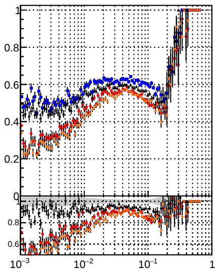
Fake rate vs \epsilon Legend: DOM CKE DOM mKEit DOM BDT DOM CKEit DOM mKEit DOM CKEit
