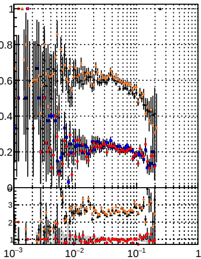
Fake rate vs \epsilon Legend: DOM CKE DOM mKEit DOM BDT BDT mKEit
