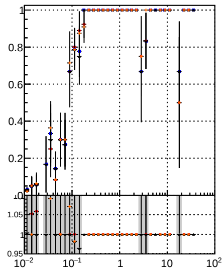
Legend for Fake rate vs vertpos: DOM CKE DOM mKEit DOM BDT DOM mKEit CKE
