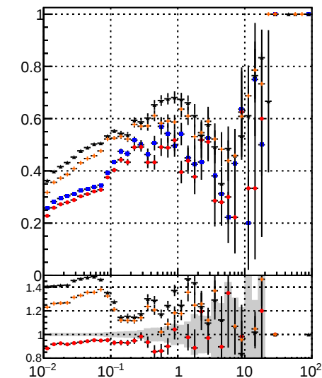
Fake rate vs \nu Legend: DOM CKE DOM mKEit DOM BDT DOM mKEit CKEit
