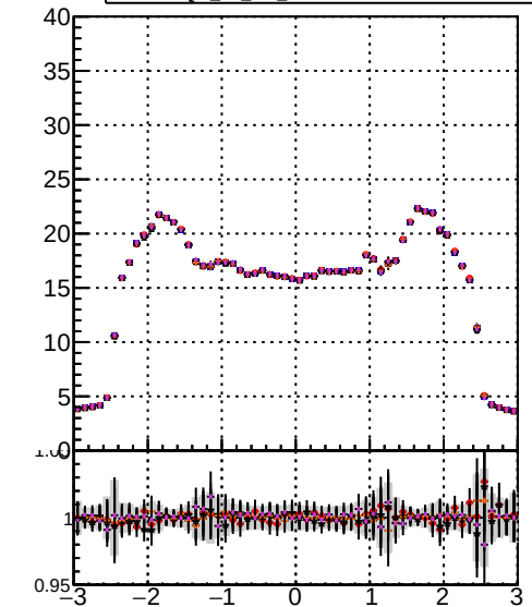
mean hit DOM TT MS init DOM TT MS thott DOM TT MS detO DOM TT MS detI
