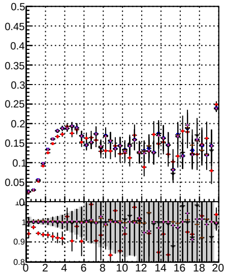
Fake rate vs. BQM TT MS LUT BQM TT MS LUT
