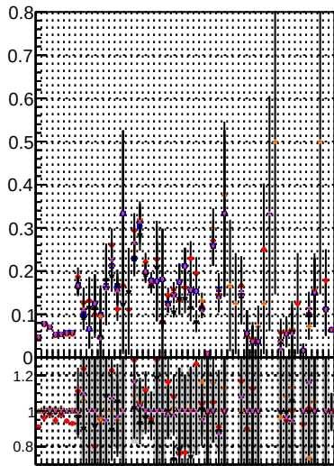
Fake rate vs. BQM TT MS LUT BQM TT MS LUT
