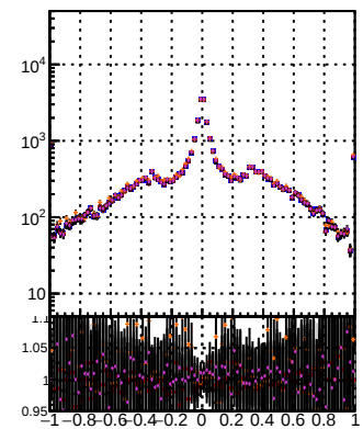
Legend for track types: \text{BOM} , \text{TT} , \text{MS} , \text{init} , \text{detr} , \text{MS}
