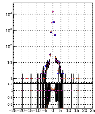
Legend for track types: \text{BOM} , \text{TT} , \text{MS} , \text{init} , \text{detr} , \text{MS}
