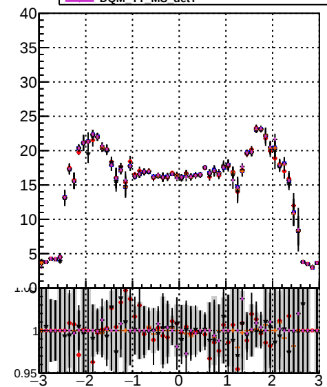
mean hit DOM TT MS DOM TT MS DOM TT MS DOM TT MS DOM TT MS DOM TT MS DOM TT MS DOM TT MS DOM TT MS DOM TT MS DOM TT MS init hptt deto deto
