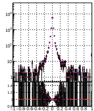
N of reco track vs dxy(PV) DQM TT MS init det DQM TT MS init det
