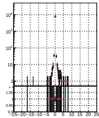
N of reco track vs dxy(PV) DQM TT MS init det DQM TT MS init det
