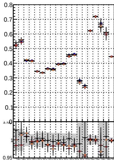
Fake rate vs. BGM noMS BGM noMS PL BGM noMS PL MS pixelLess or BGM mod MS
