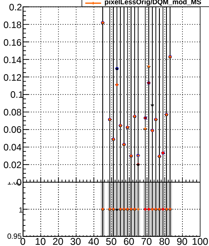
DQM_noMS DQM_moMS_PL Orig/DQM_orig_MS pixelLessOrig/DQM_mod_MS
