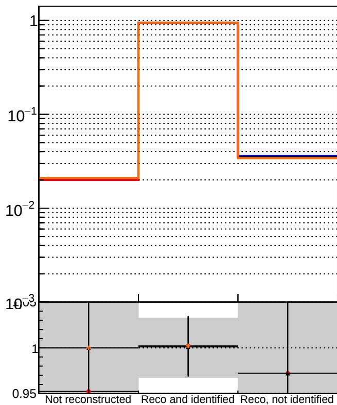
DQM_noMS DQM_moMS_PL Orig/DQM_orig_MS pixelLessOrig/DQM_mod_MS
